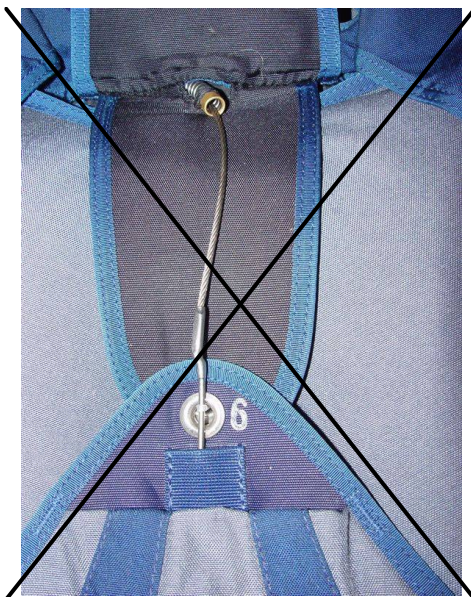
Stávající způsob balení. Pořadí balení chlopní záložního padáku 1-2-3-4-5-6. Nahrazeno novým způsobem balení.
