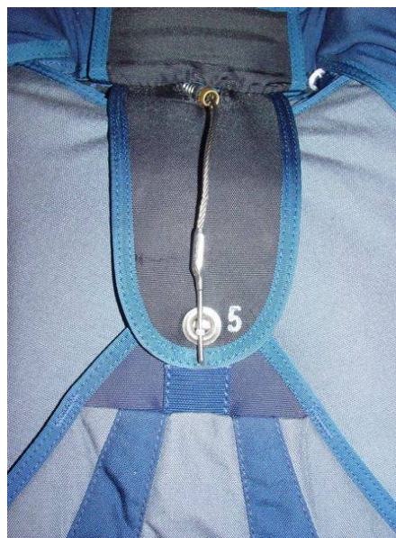
Nový způsob balení. Pořadí balení chlopní záložního padáku 1-2-3-4- 6-5 .
